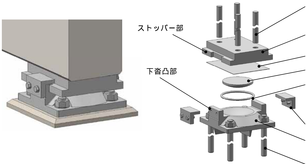
図 1 高力黄銅支承板支承の構造図
