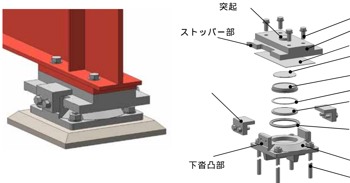
図2 BP.B 支承レベル1 地震動支持型の構造図
