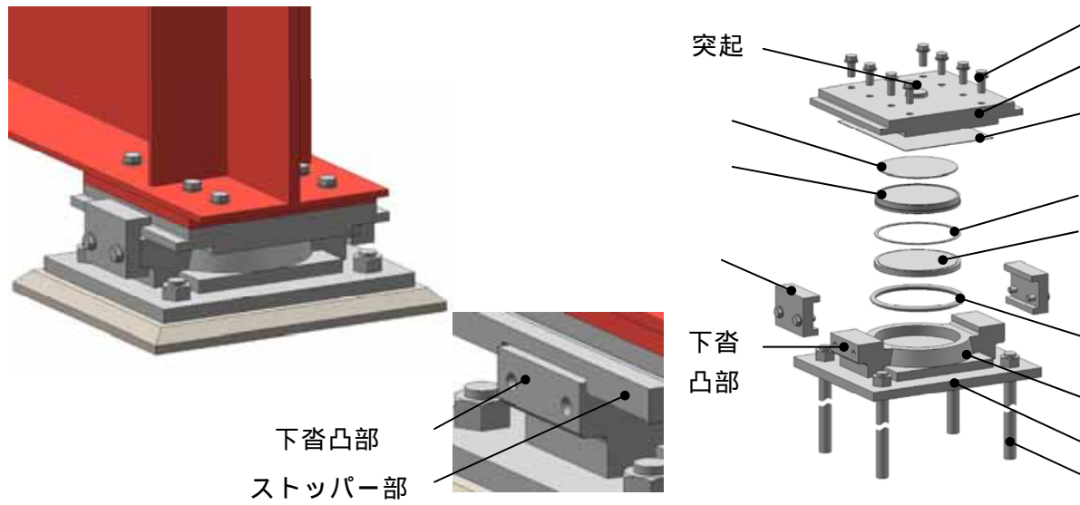
図3 BP.B 支承レベル2 地震動支持型の構造図
