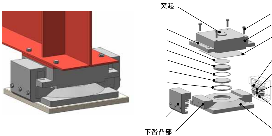
図 5 BP.B 支承負反力支持型の構造図
