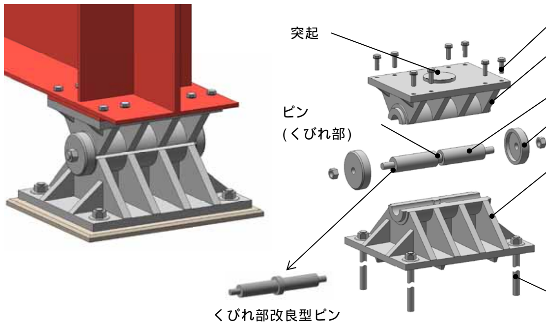
図6 ピン支承支圧型の構造図
