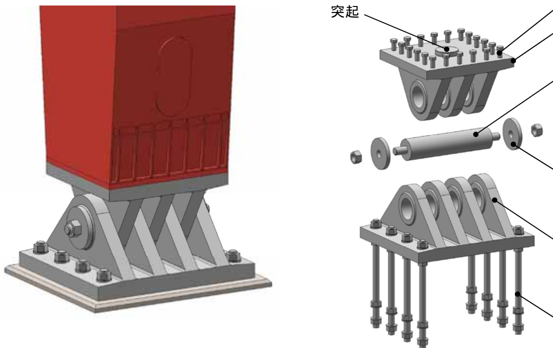
図7 ピン支承せん断型の構造図
