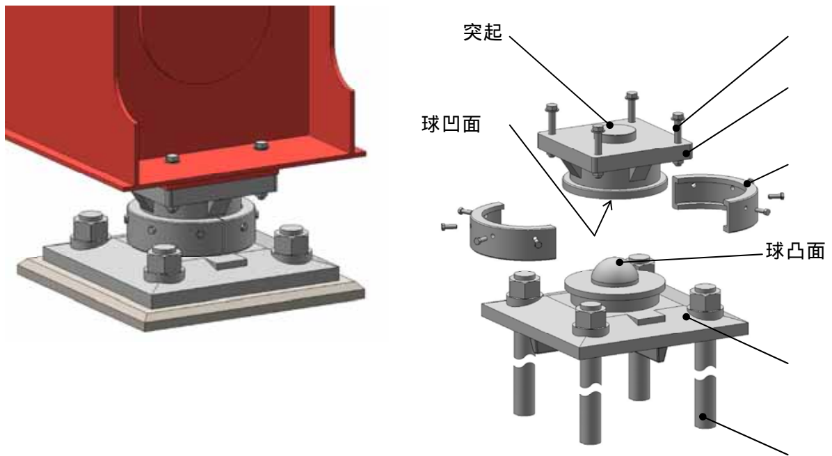
図 8 ピボット支承の構造図
