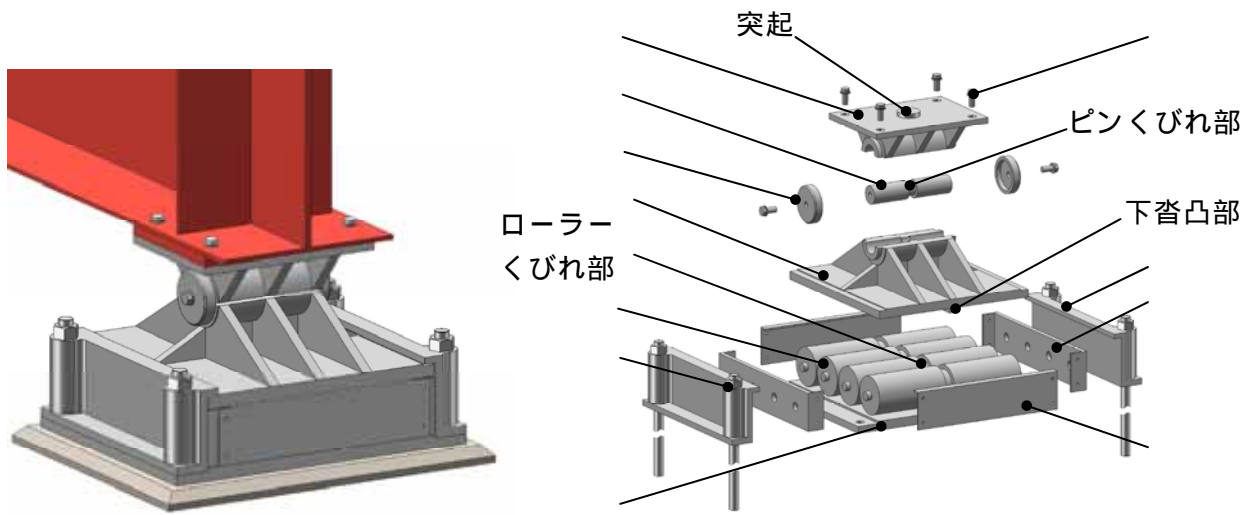
図9 普通鋼ピンローラー型支承の構造図
