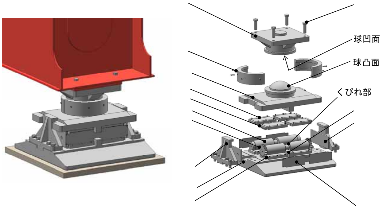
図 12 ピボットローラー支承の構造図
