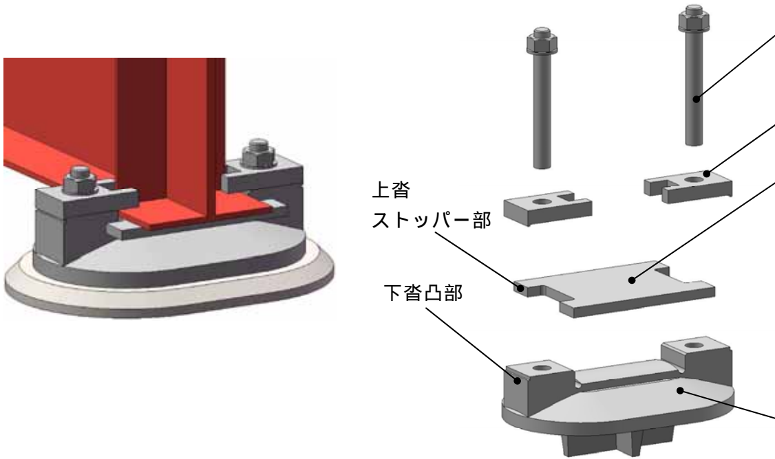
図 13 線支承の構造図
