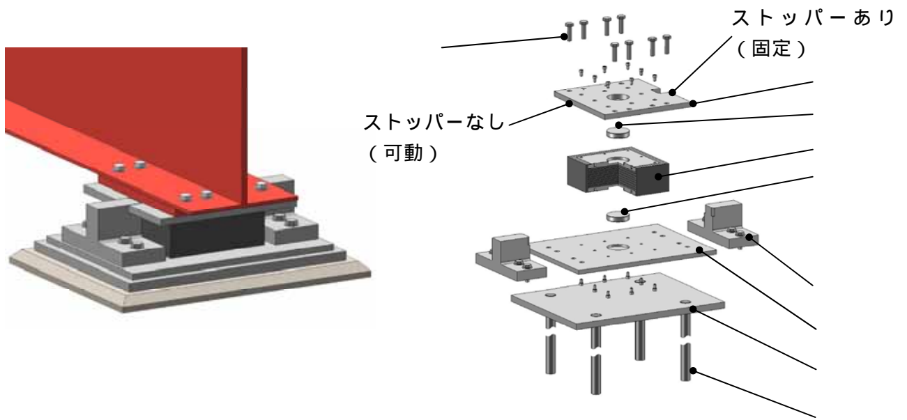
図 1.15 ゴム支承せん断型の構造図
