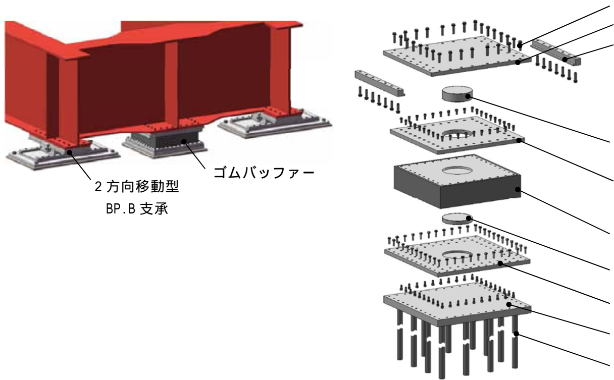
図 1.17 機能分離型支承バッファー横置き型の構造図
