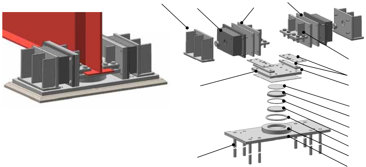
図 1.18 機能分離型支承バッファ縦置き型の構造図
